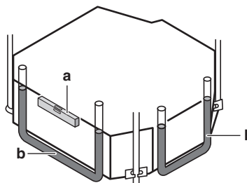
Рис. 4.2: Проверьте выравнивание агрегата
