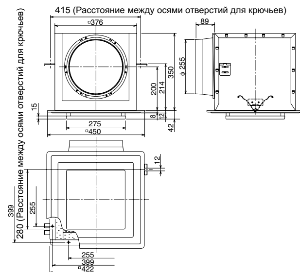
K-DGL250A
